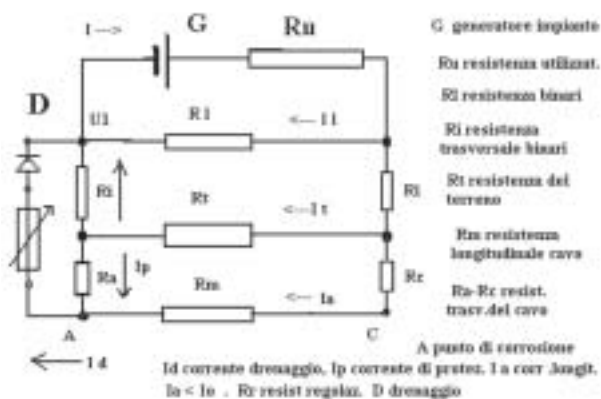
Schema elettrico di circuito di inserzione di alimentatore catodico
