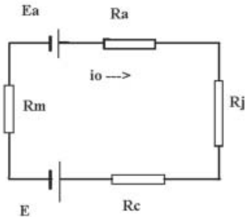
Circuito equivalente di un processo di corrosione elettrochimica.
