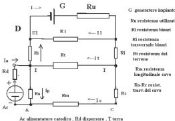
Circuito elettrico di inserzione di un drenaggio unidirezionale.
