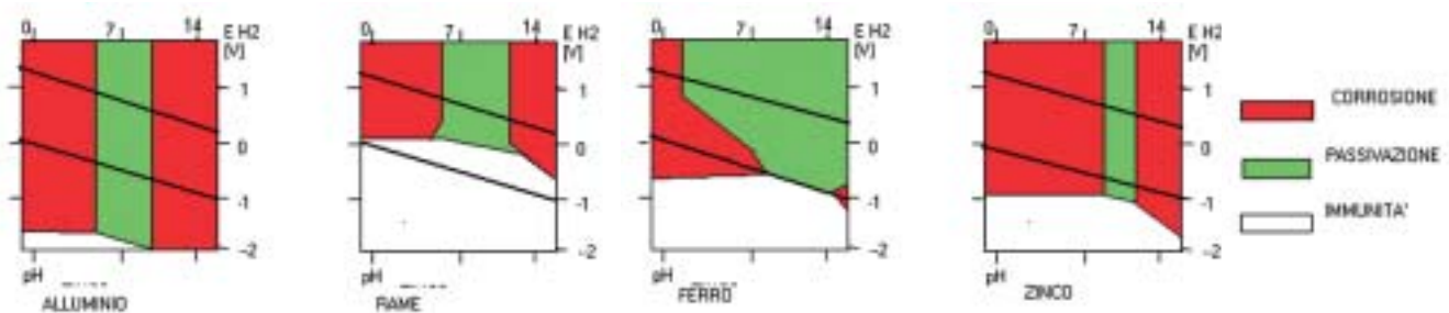
Diagrammi di Pourbaix
