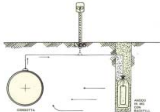
Inserzione di un anodo reattivo
